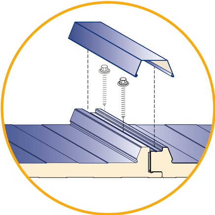
Detalle de solape. Usar 2 tornillos en vanos superiores a 2,00 m.
